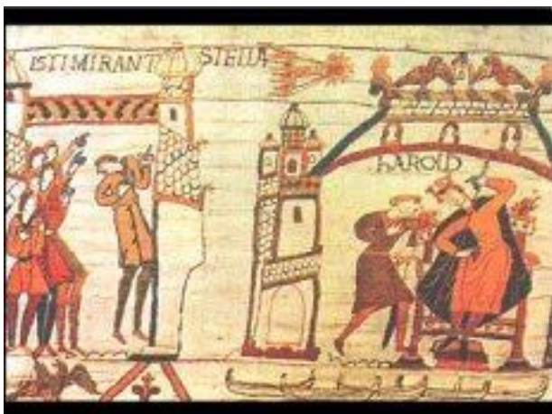
Изображение кометы Галлея в 1066 года на гобелене из Байё
