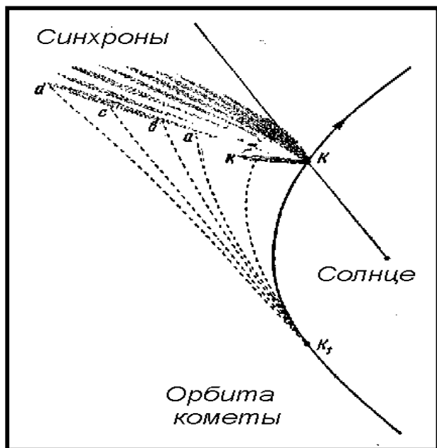
Рис. 4. Если из ядра кометы будут в один момент времени выброшены частицы с различными скоростями, то через некоторое время они образуют синхроны. [ С.В. Орлов, «О природе комет», 1960]
