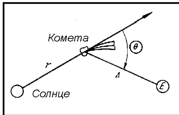
Рис. 3. Изменение блеска кометы происходит из-за того, что меняется расстояние \Delta между ней и Землей, r между ней и Солнцем
