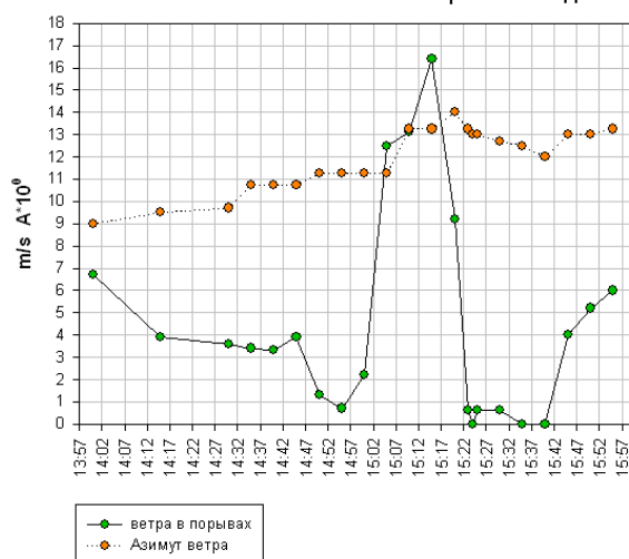
Направление и скорость ветра. Полное солнечное затмение 29 марта 2006 год.
