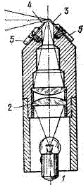
Рис. 53. Осветительная система хорошо оборудованного теневого прибора: 1 — лампа, 2 — конденсор, 3 — нож, 4 — вторая щечка щели, 5 — прижимная пластина
