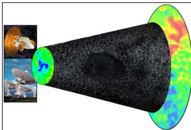
В направлении на новообнаруженное гигантское "отверстие" в космосе спутник WMAP (фото слева вверху) видит "холодное пятно", в то время как VLA (фото слева внизу) видит меньшее количество радиогалактик. Изображение: Bill Saxton, NRAO/AUI/NSF, NASA с сайта www.nrao.edu .
