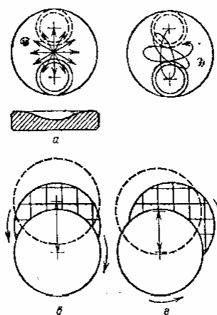
Рис. 33. Обдирка и шлифовка зеркала: а — обдирка кольцом через центр и поверхность, которая при этом получается, б — обдирка эллиптическим штрихом для устранения этого недостатка, в — обработка шлифовальником через центр, г — то же по хорде.
