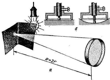
Рис. 34. Определение радиуса кривизны мокрого зеркала с лампой (а) и стрелки кривизны сферометром (б)
