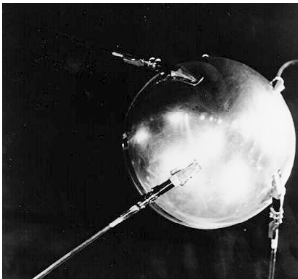
Первопроходец Вселенной.
