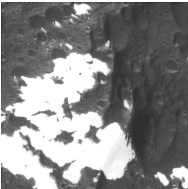
Ландшафты Япета.
